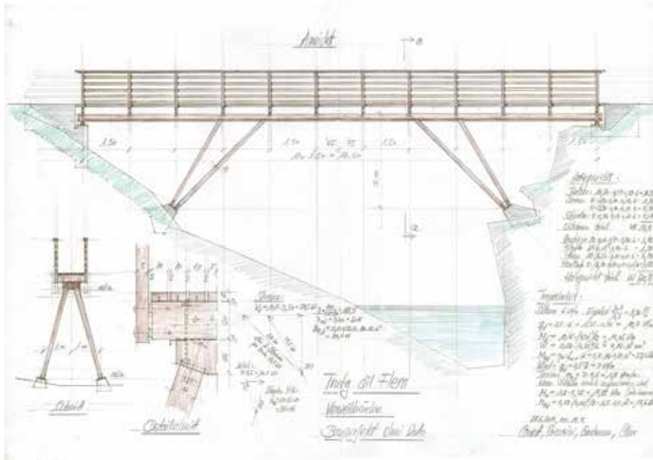
Dessin constructif du pont, Trug dil Flem, 2010 (© JÜRIG CONZETT)
